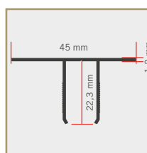
STAFFA DI FISSAGGIO GUIDA LATERALE (PER FISSAGGI LATERALI)
