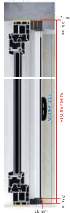
FISSAGGIO LATERALE
