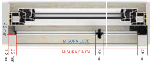
FISSAGGIO LATERALE
