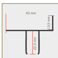
STAFFA DI FISSAGGIO RISCOSTRO A MURO E GUIDA SUPERIORE (PER FISSAGGI FRONTALI)
