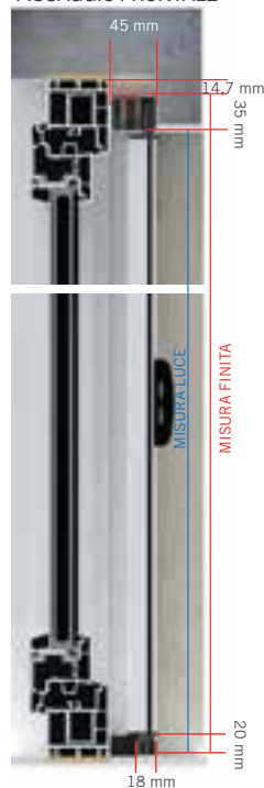
FISSAGGIO FRONTALE
