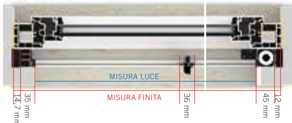
FISSAGGIO FRONTALE
