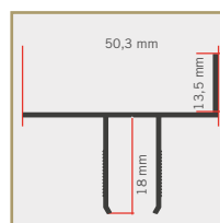
STAFFA DI FISSAGGIO GUIDA LATERALE (DI SERIE, PER FISSAGGI FRONTALI)
