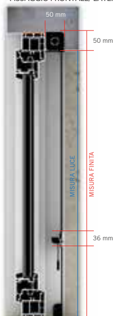
FISSAGGIO FRONTALE/ LATERALE
