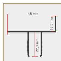
STAFFA DI FISSAGGIO RISCONTRO A MURO E GUIDA SUPERIORE (DI SERIE, PER FISSAGGI FRONTALI)
